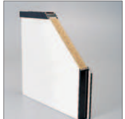
Schnitt Typen RW und VB
